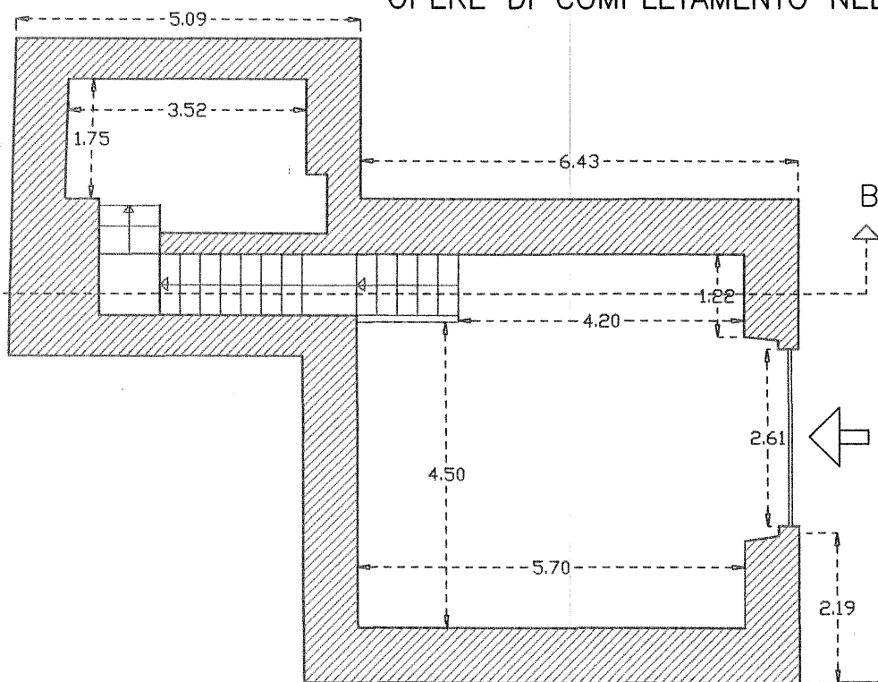
PIANTA LOCALI PARROCCHIALI — SCALA 1: 100
