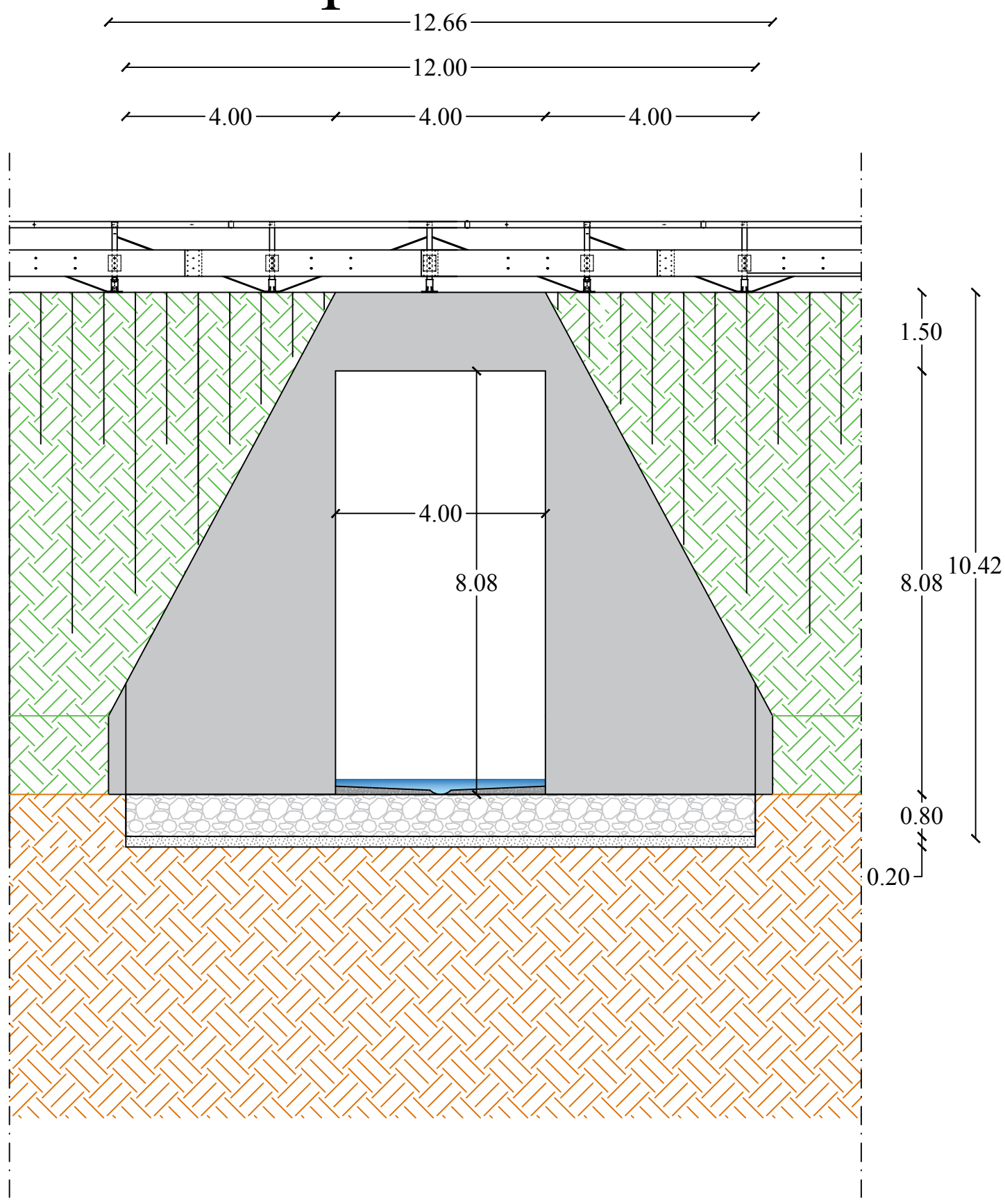
Prospetto Laterale
