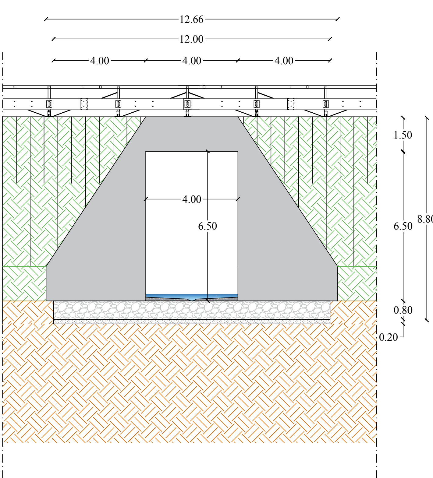
Prospetto Laterale
