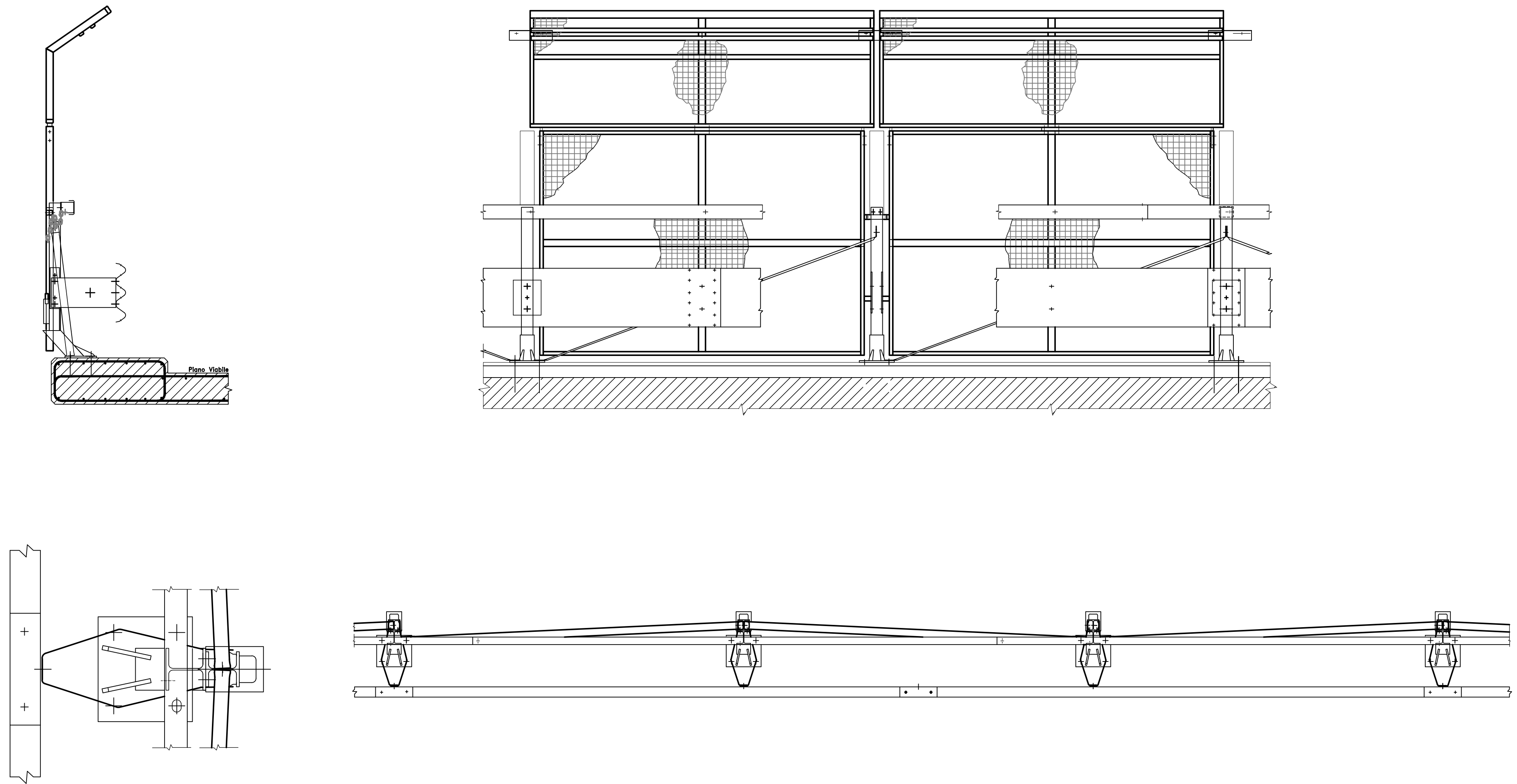
PARTICOLARI GUARDARAIL scala 1:25
