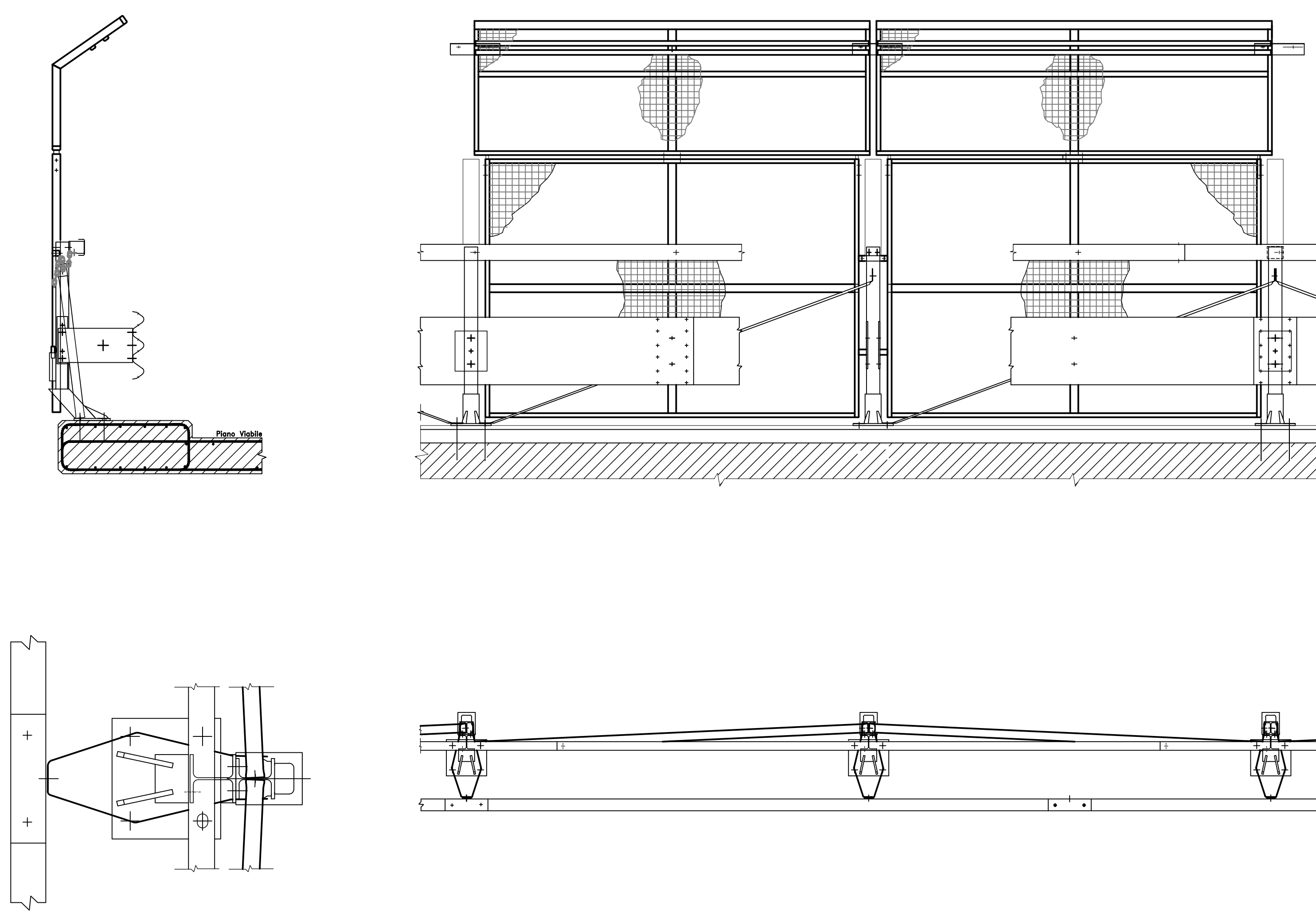
PARTICOLARI GUARDARAIL scala 1:25
