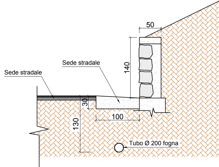
SEZIONE 1 Scala 1 : 50
