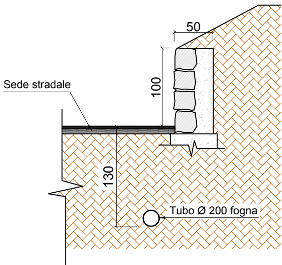
SEZIONE 3 Scala 1 : 50
