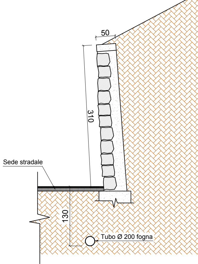
SEZIONE 2 Scala 1 : 50
