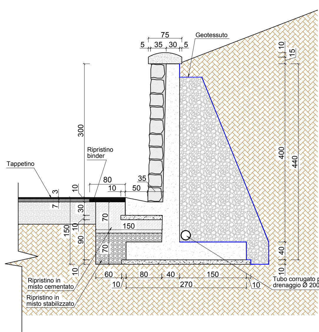
MURO TIPO SEZIONE 2 Scala 1 : 50
