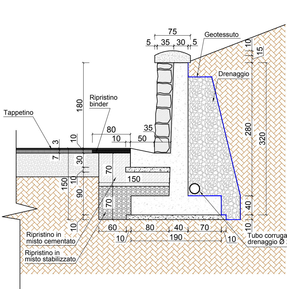
MURO TIPO SEZIONE 1 Scala 1 : 50
