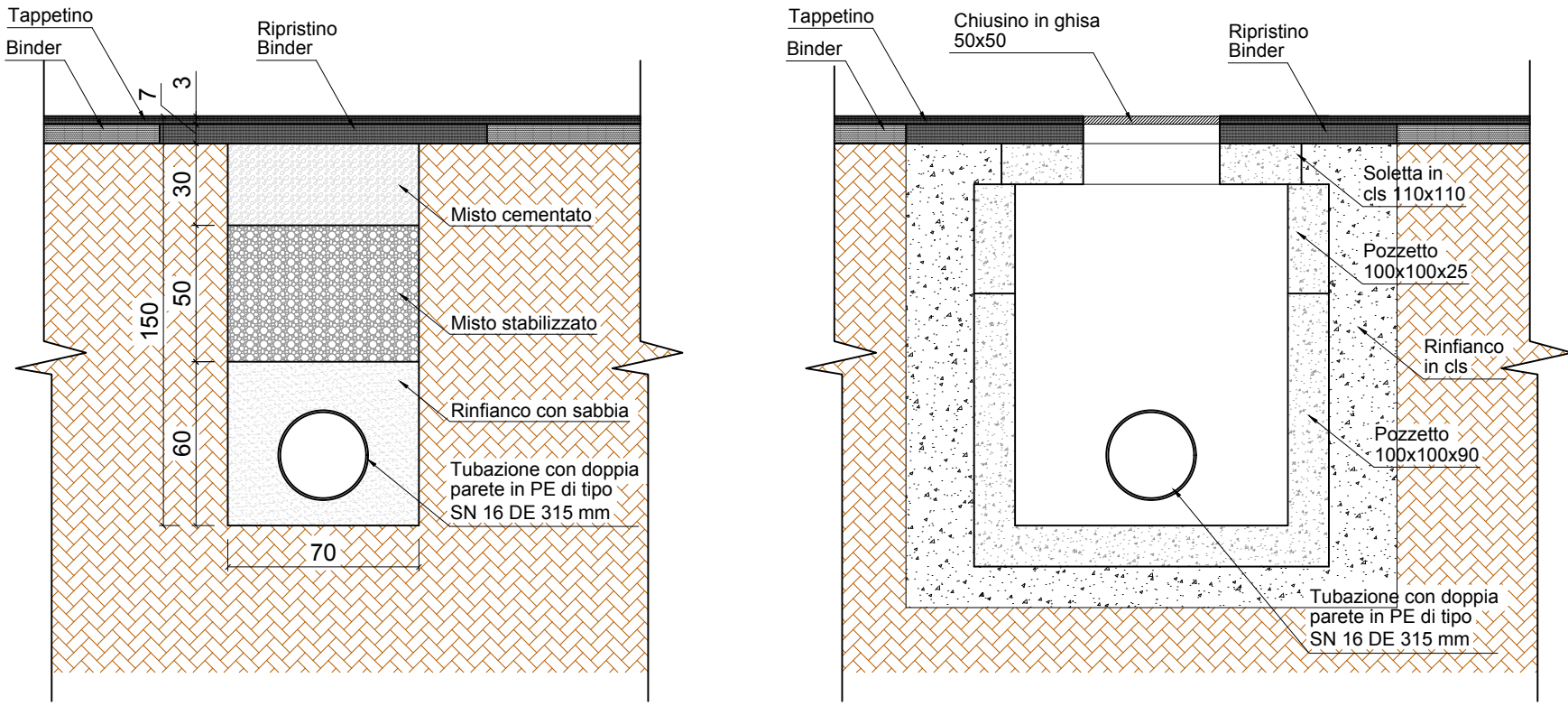
SEZIONE SCAVO FOGNA E POZZETTO Scala 1 : 25
