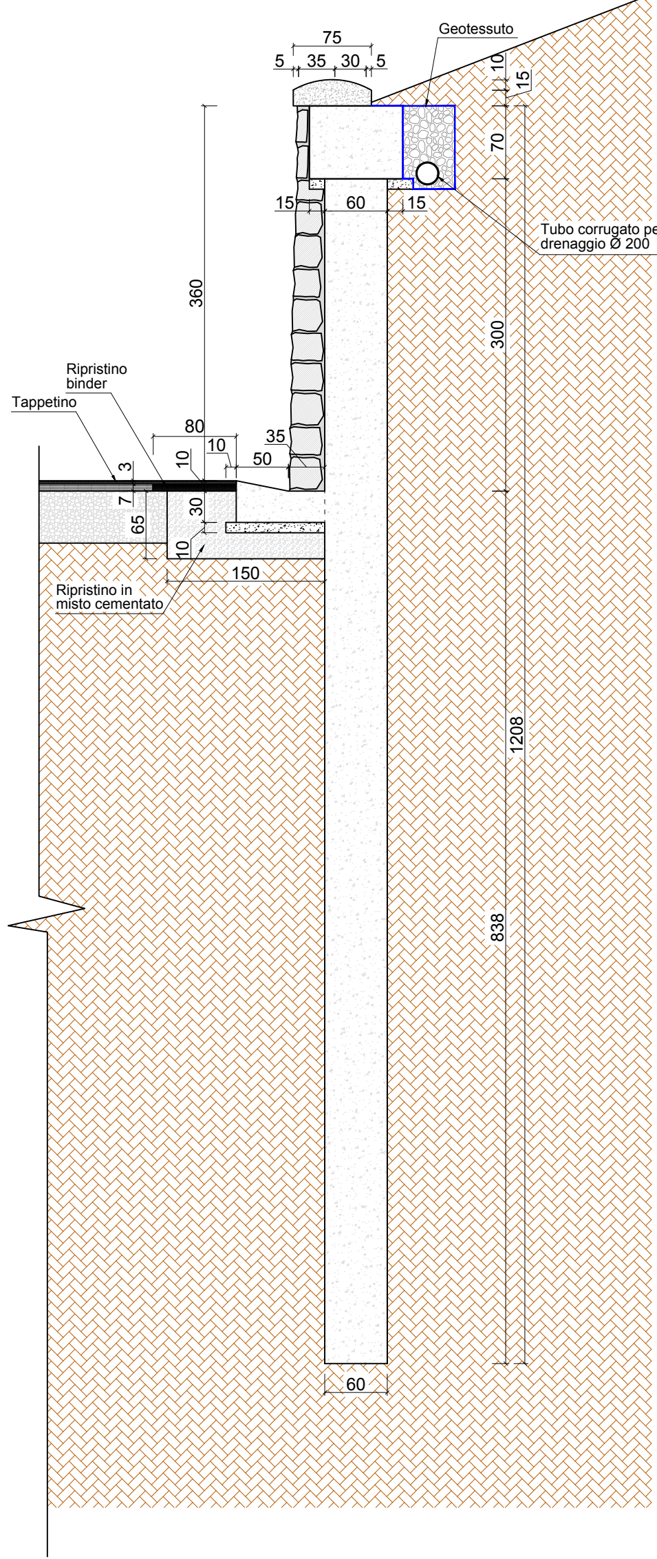
SEZIONE PALIFICATA Scala 1 : 50
