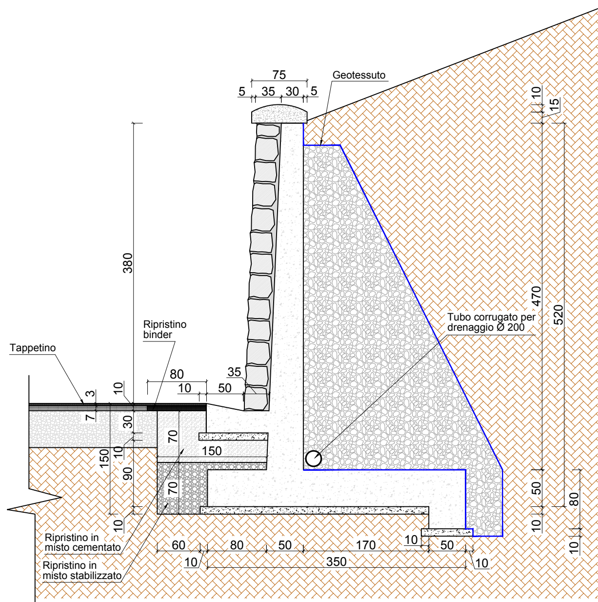
MURO TIPO SEZIONE 3 Scala 1 : 50
