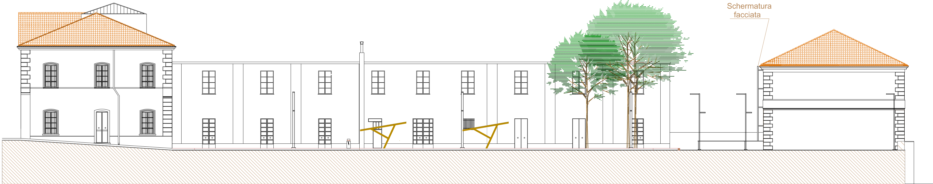
PROFILO B-B
